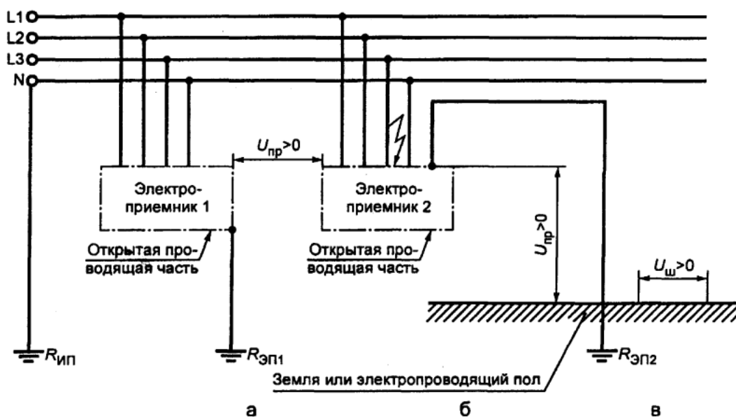
Рисунок В.10 — Сеть ТТ с нулевым рабочим проводником с однофазным замыканием на корпус
